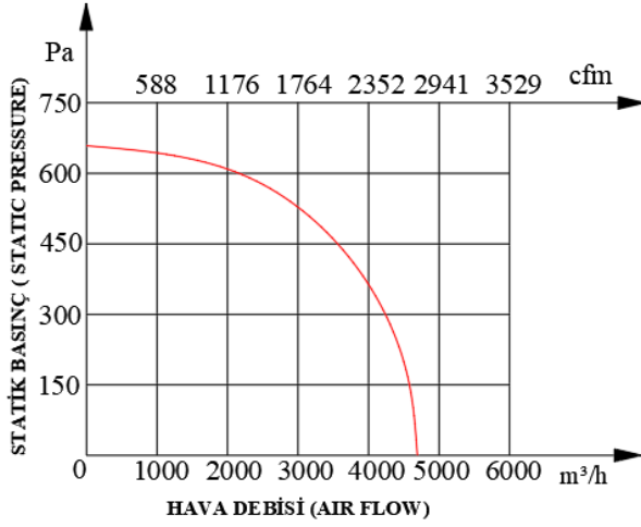
DKFH 400
