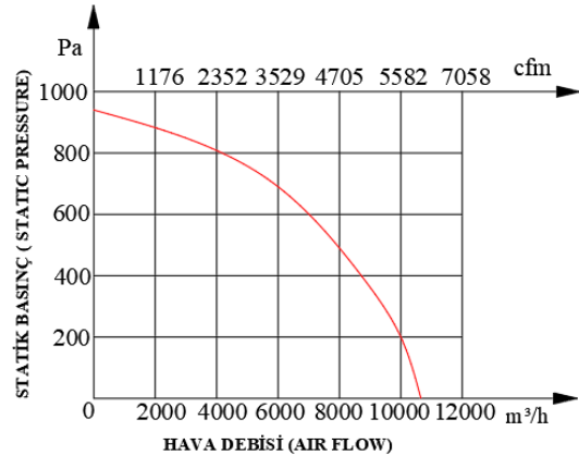
DKFH 560
