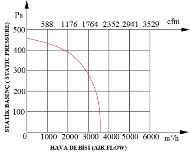
DKFH 355
